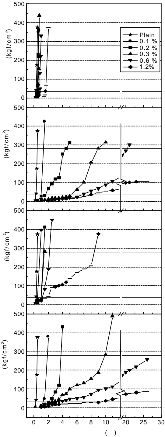
<그림-5> 응결지연성 혼화제의 혼입률 변화에 따른 응결시간
