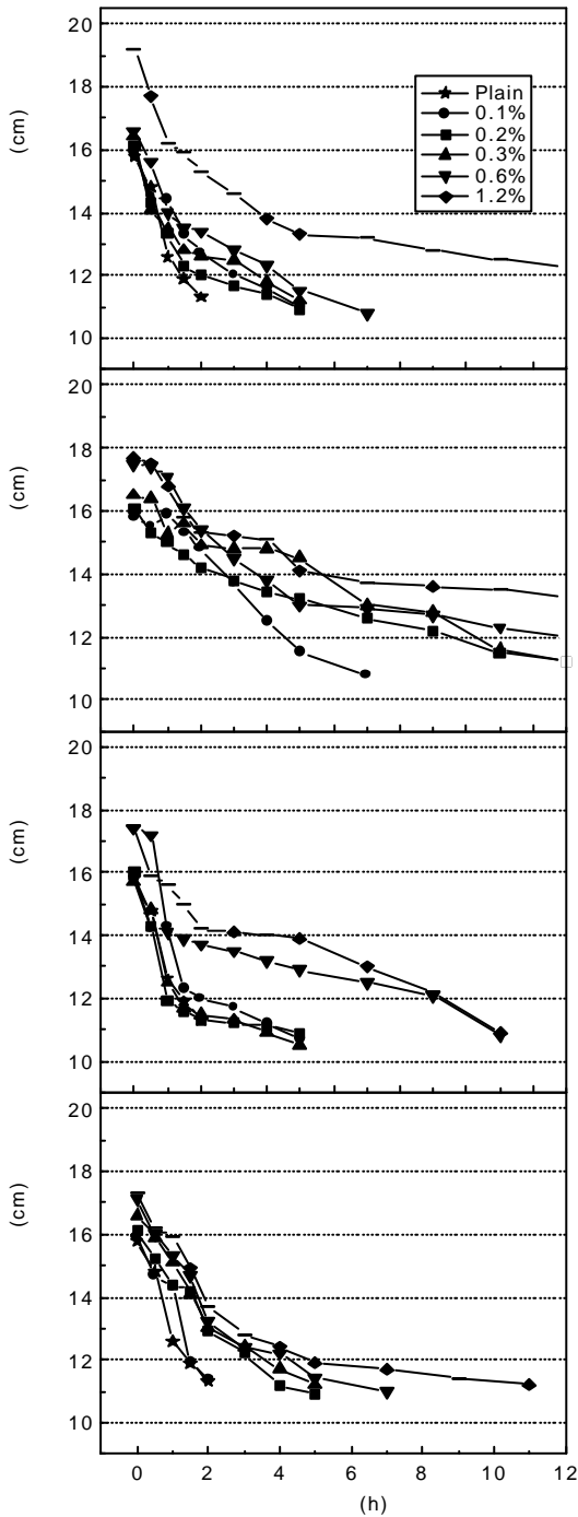
<그림-4> 응결지연성 혼화제의 종류와 혼입률 변화에 따른 플로우 결시변화
