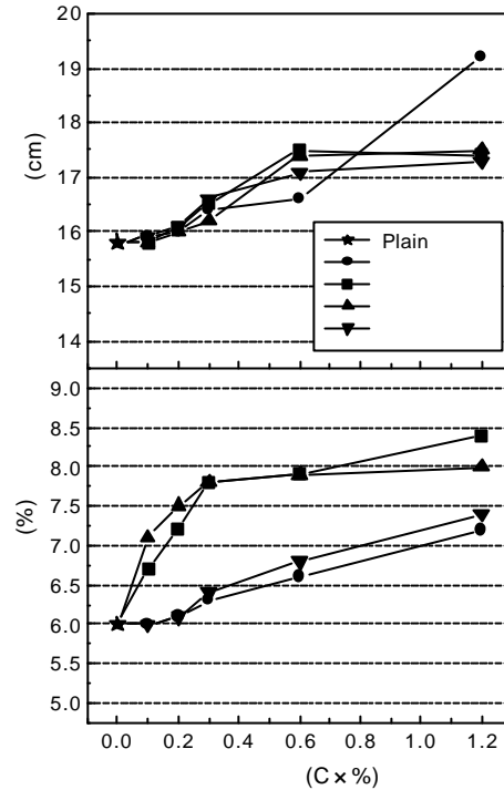
<그림-3> 응결지연성 훈화제의 혼입률 변화에 따른 플로우 값과 공기량
