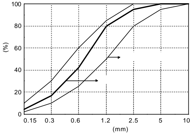
<그림-1> 골재의 입도 곡선
